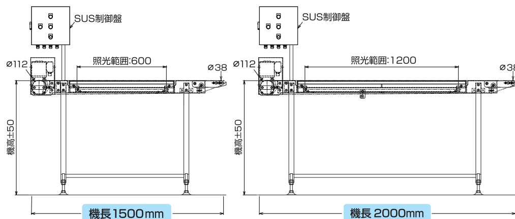
寸法図
